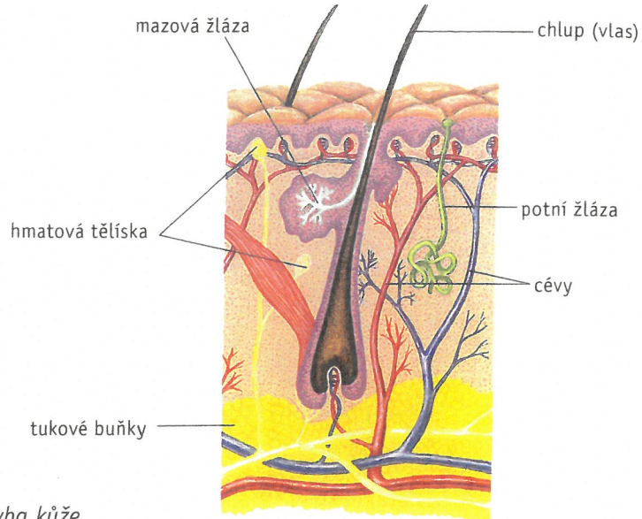
Stavba kůže
